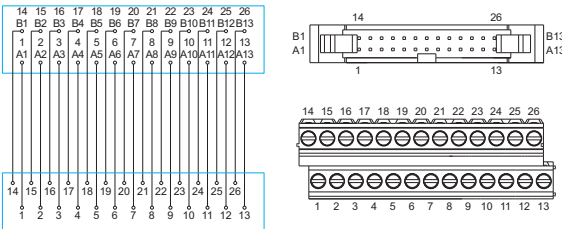
DM72-IDC-26-26-4Y-00Z(H) DM50-IDC-26-26-4Y-00Z(H)
