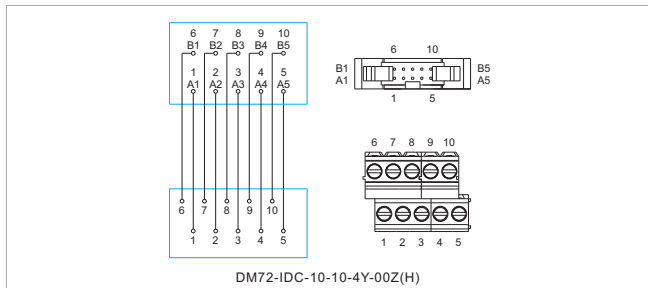
DM72-IDC-10-10-4Y-00Z(H)
