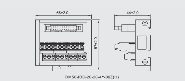
DM50-IDC-20-20-4Y-00Z(H)
