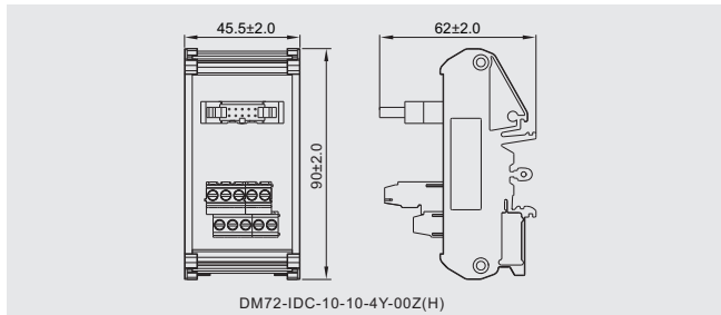
DM72-IDC-10-10-4Y-00Z(H)
