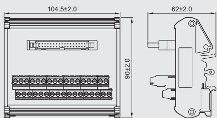
DM72-IDC-34-34-4Y-00Z(H)
