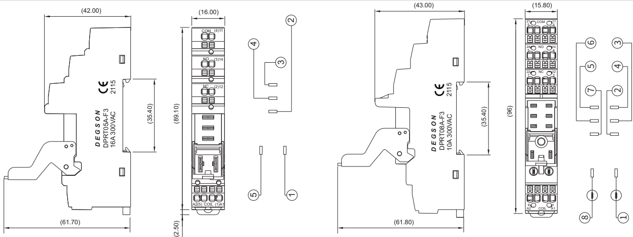
DPRT05A-F3
