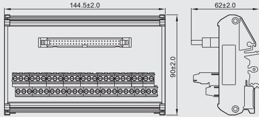
DM72-IDC-50-50-4Y-00Z(H)
