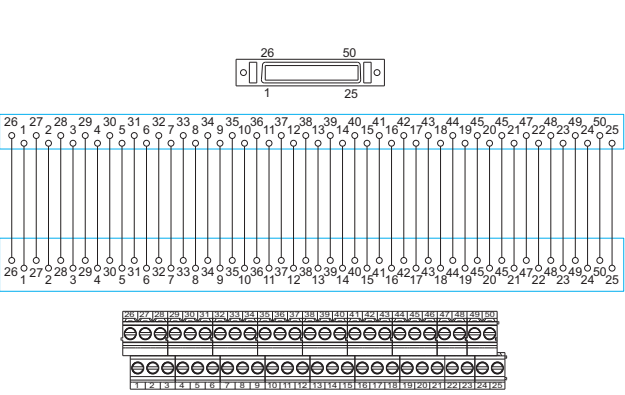
DM50-MDR-50-50-4Y-00Z(H)
