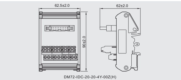
DM72-IDC-20-20-4Y-00Z(H)
