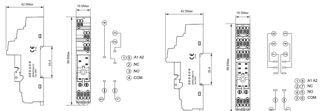
DPRC05A-F3
