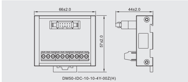
DM50-IDC-10-10-4Y-00Z(H)
