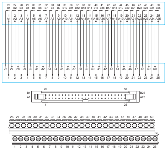
DM72-IDC-50-50-4Y-00Z(H) DM50-IDC-50-50-4Y-00Z(H)
