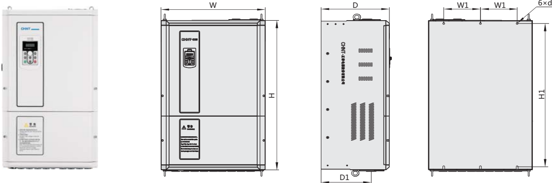
NVF2G-75/TS4 – NVF2G-315/PS4A
