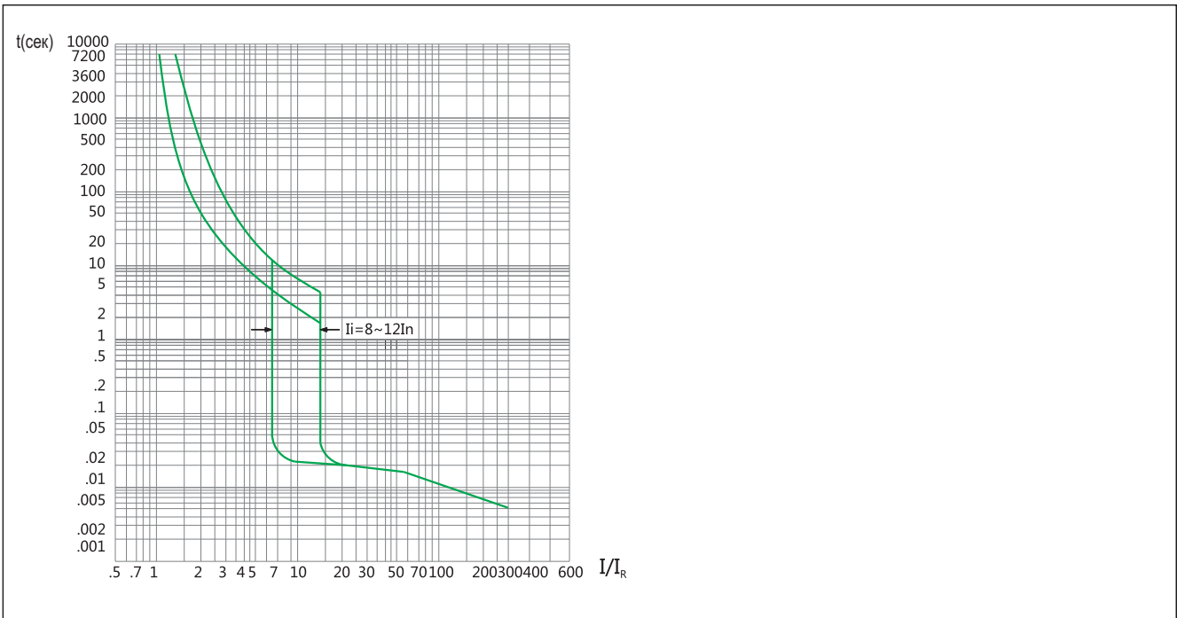
NM8-250(100A~250A)
