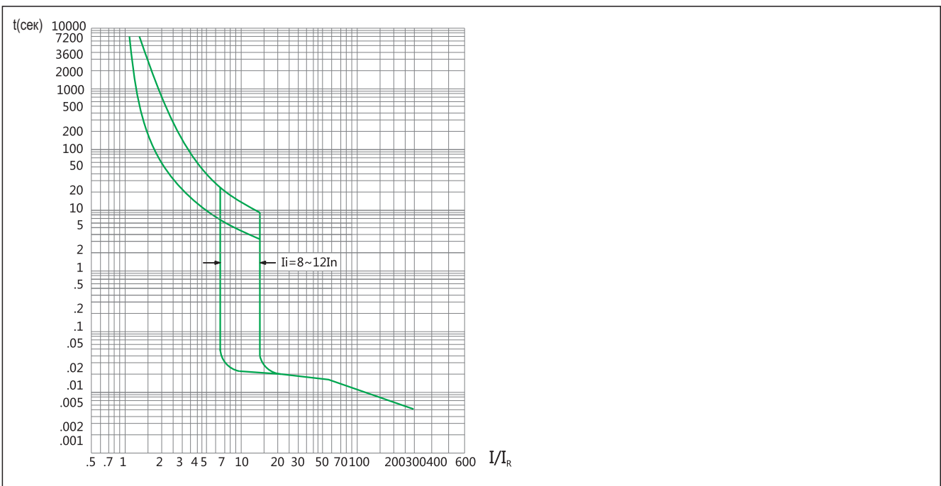
NM8-400,630(250A~500A)
