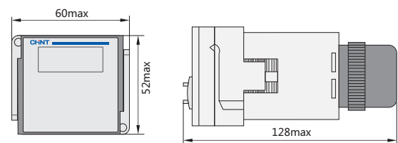
Профильные установочные размеры изделий серии JSS48B
