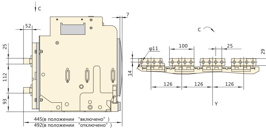
NA8G-3200(I n =2900, 3200A) выдвижное исполнение ,заднее присоединение, горизонтальные контактные пластины
